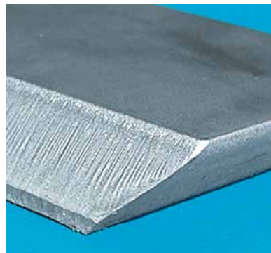
Fasenbeispiel in Baustahl: 15 mm 45° YDS und 30° VAS (Schneidqualität abhängig von Material)
